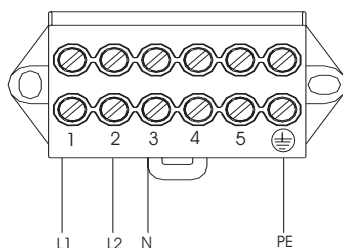
230V, 2N ~
