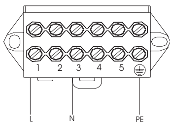
230V~
